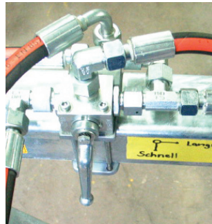
Ventil Schnell- / Langsamlauf
